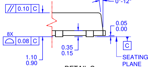
DETAIL C SCALE: 2:1
