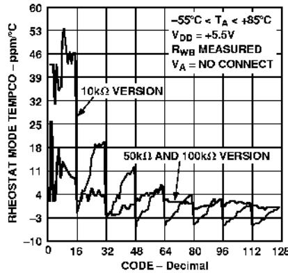
Figure 14. \Delta R_{WB}/\Delta T Rheostat
