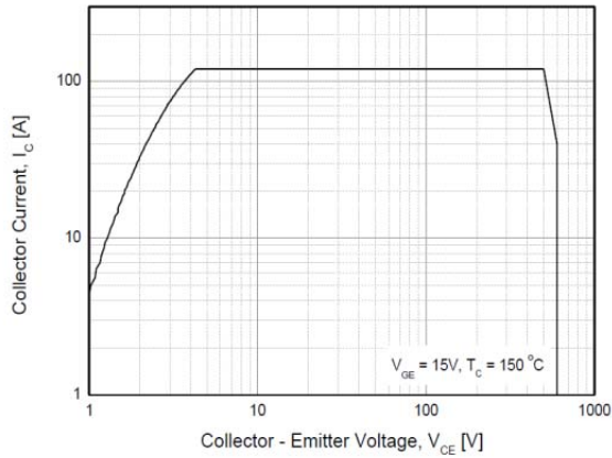
Fig. 15 RBSOA
