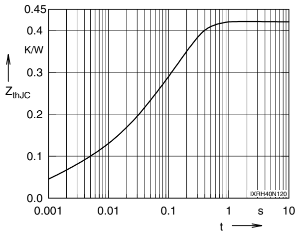
Fig. 16 Typ. transient thermal impedance
